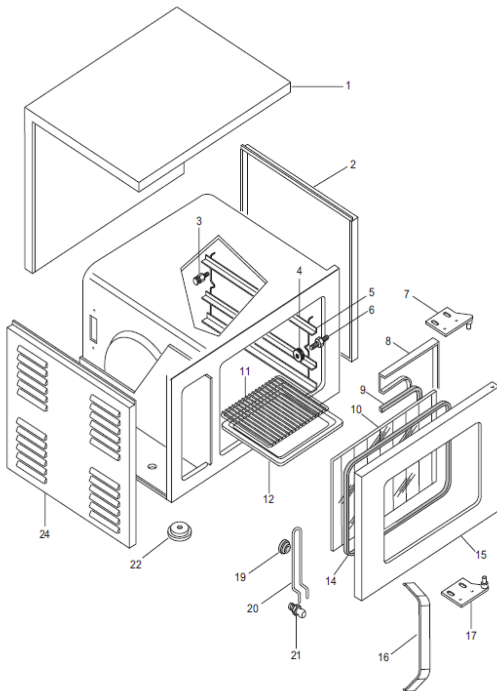
3 GN 2/3 ELECTRIC CONVECTION OVEN FORNO CONVEZIONE ELETTRICO 3 GN 2/3
